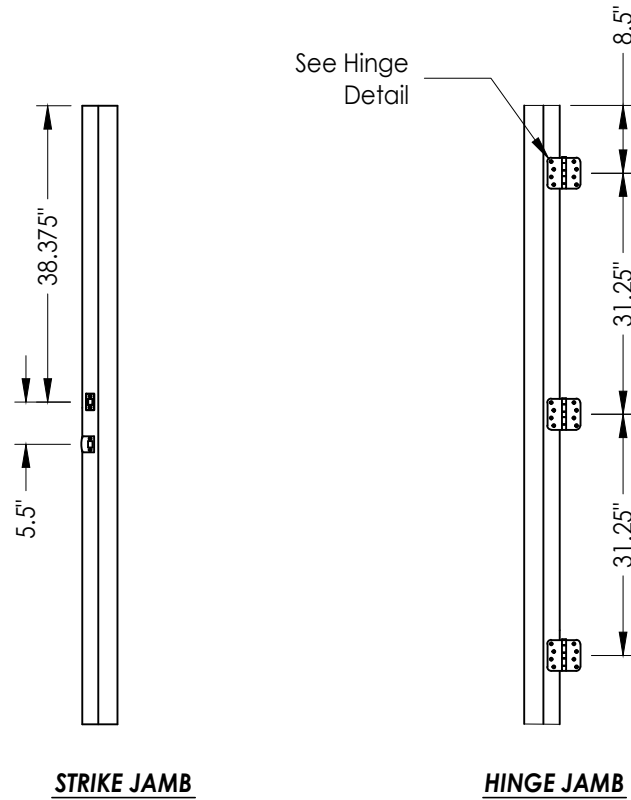
STRIKE JAMB
