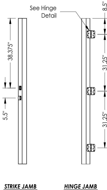
STRIKE JAMB
